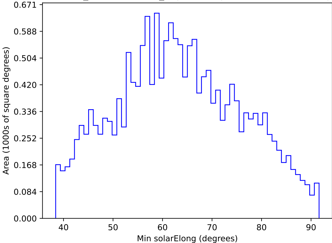
weather_cloudso20v3.4_10yrs WFD y band: Min solarElong
