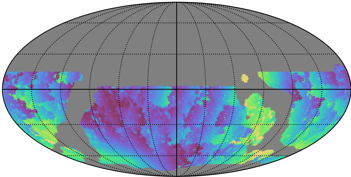
weather_cloudso20v3.4_10yrs WFD u band: Min solarElong
