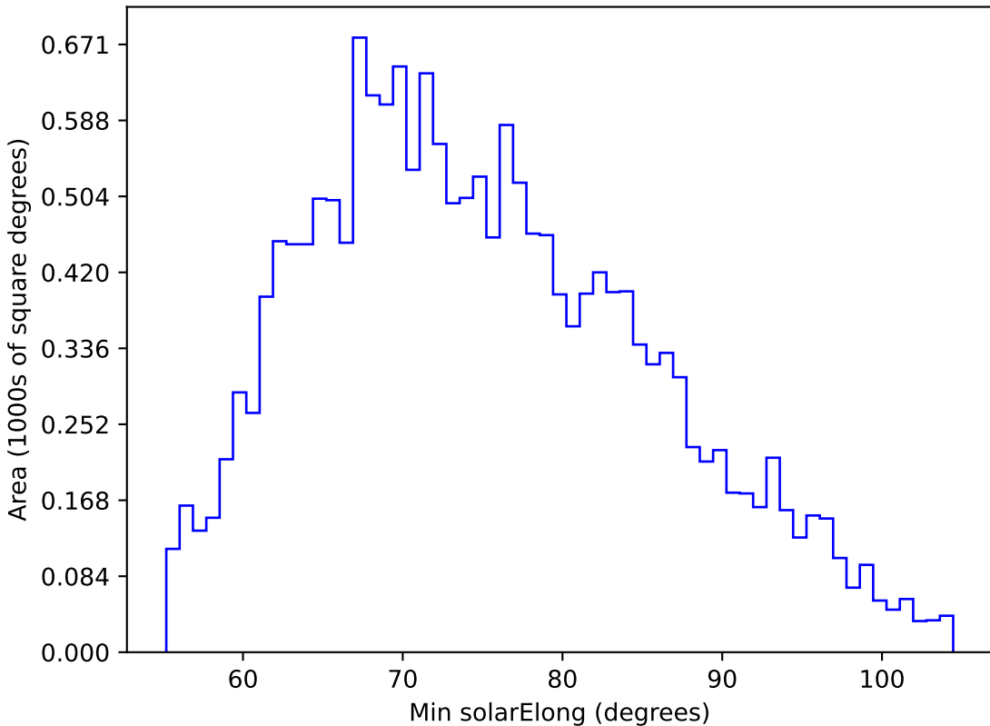
weather_cloudso20v3.4_10yrs WFD u band: Min solarElong
