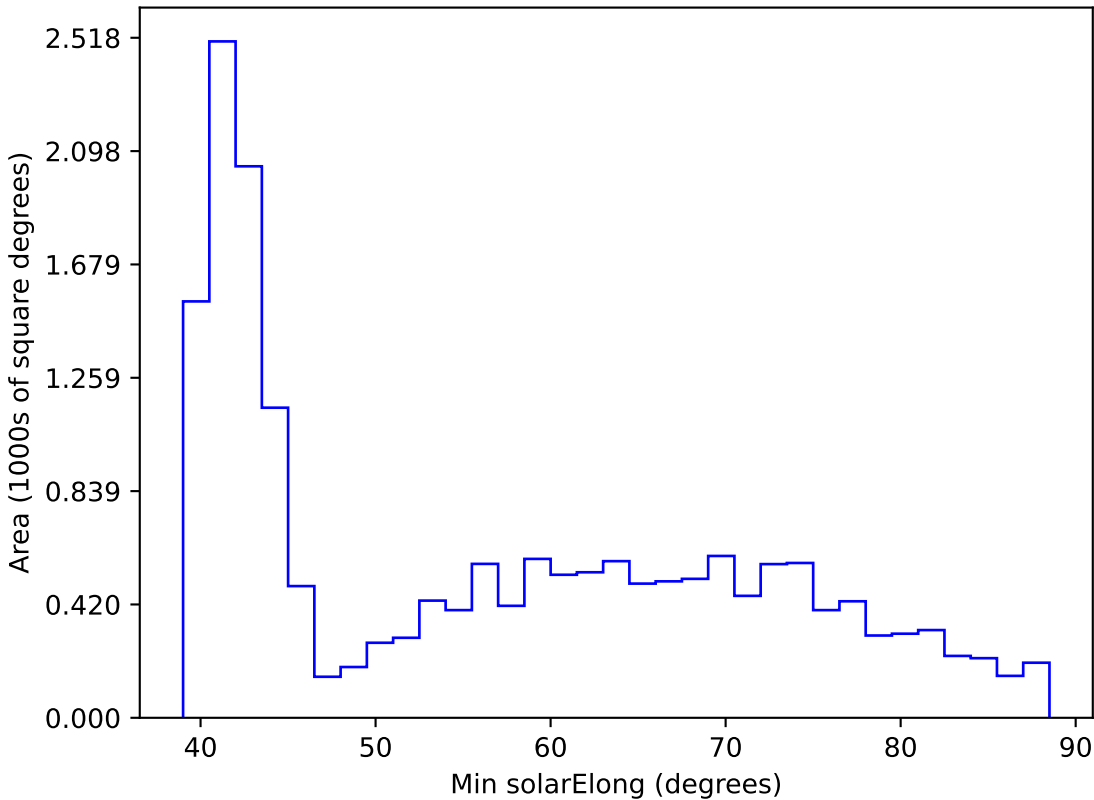
weather_cloudso20v3.4_10yrs WFD r band: Min solarElong
