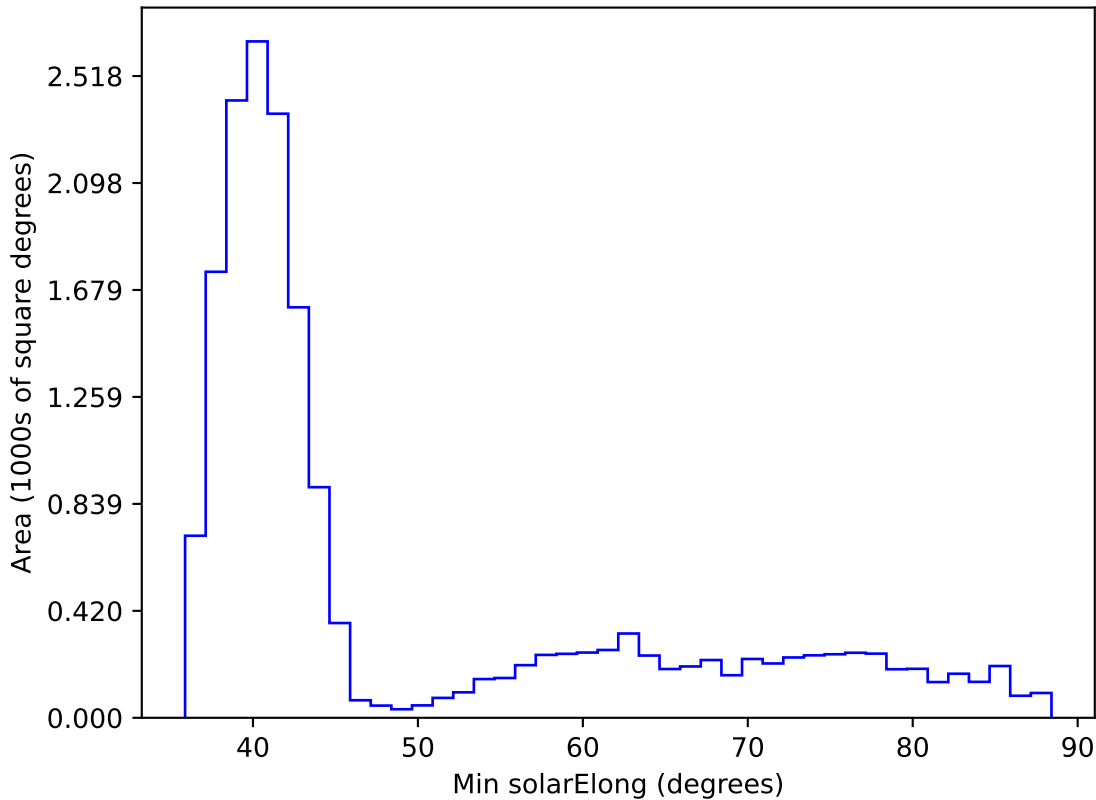
weather_cloudso20v3.4_10yrs WFD i band: Min solarElong
