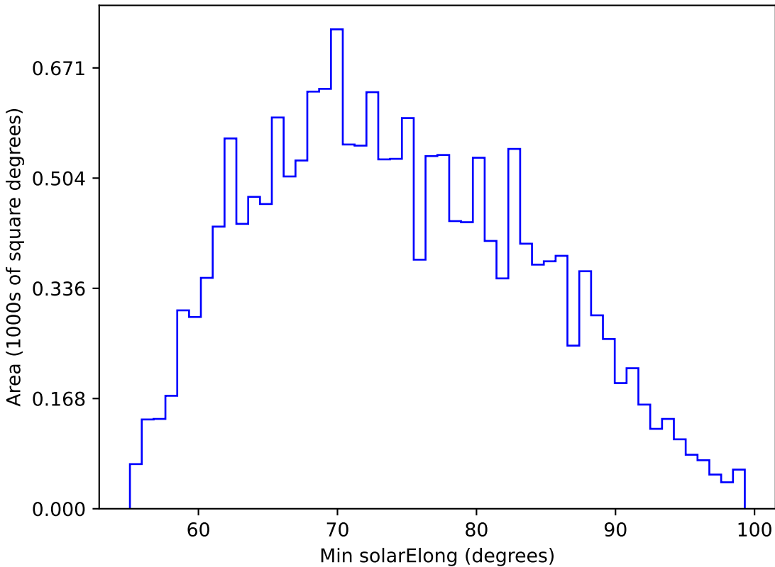
weather_cloudso20v3.4_10yrs WFD g band: Min solarElong
