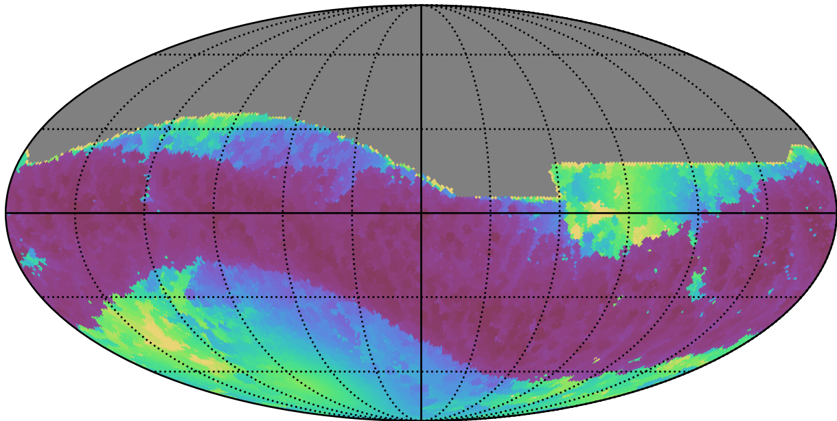
weather_cloudso20v3.4_10yrs All sky z band: Min solarElong
