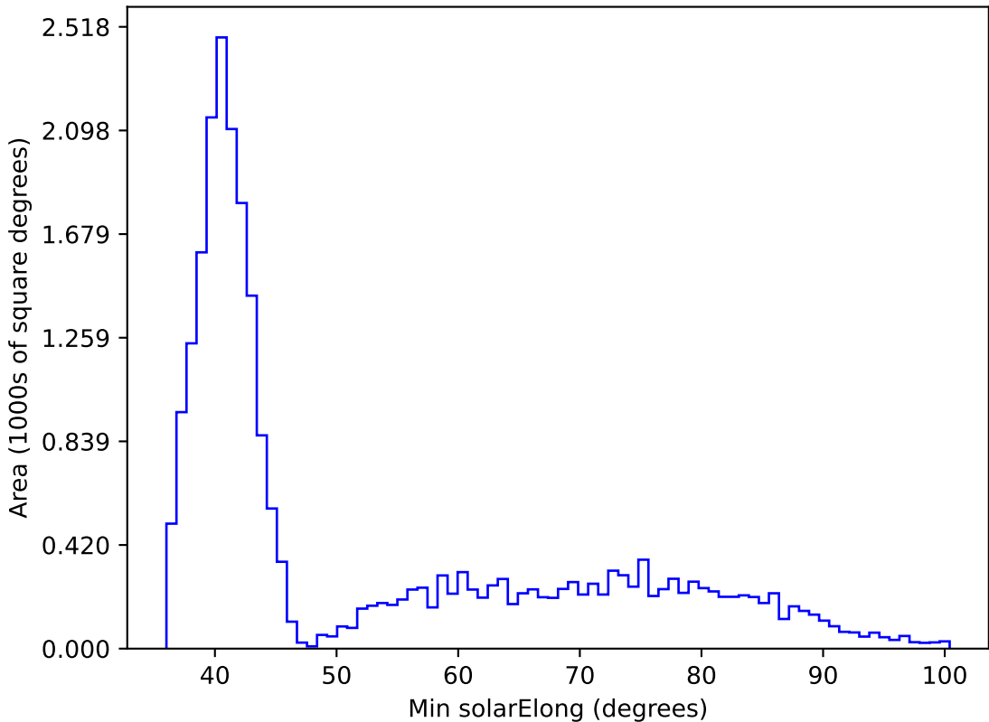
weather_cloudso20v3.4_10yrs All sky z band: Min solarElong
