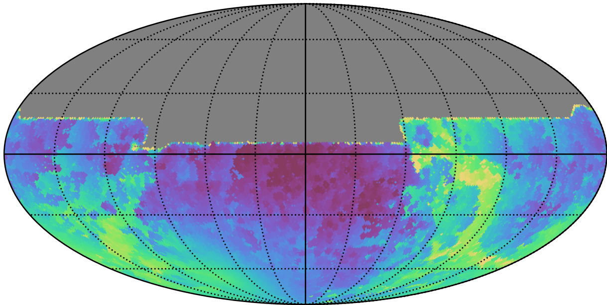
weather_cloudso20v3.4_10yrs All sky y band: Min solarElong
