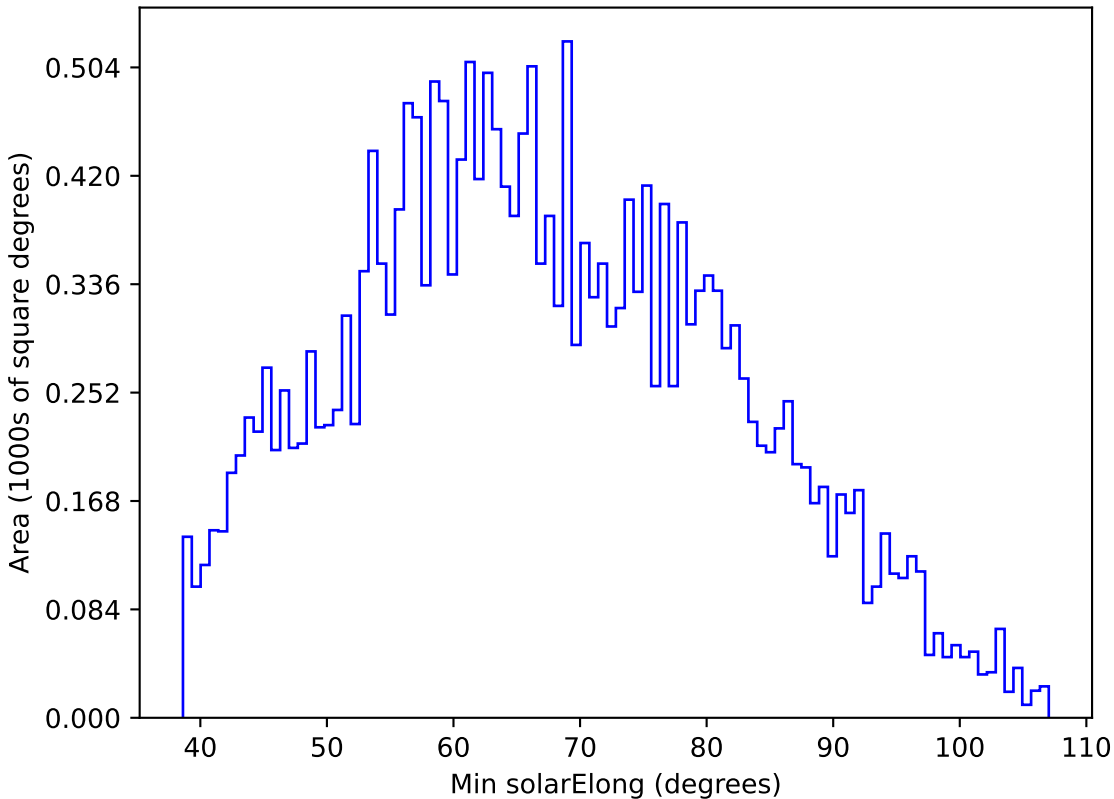
weather_cloudso20v3.4_10yrs All sky y band: Min solarElong
