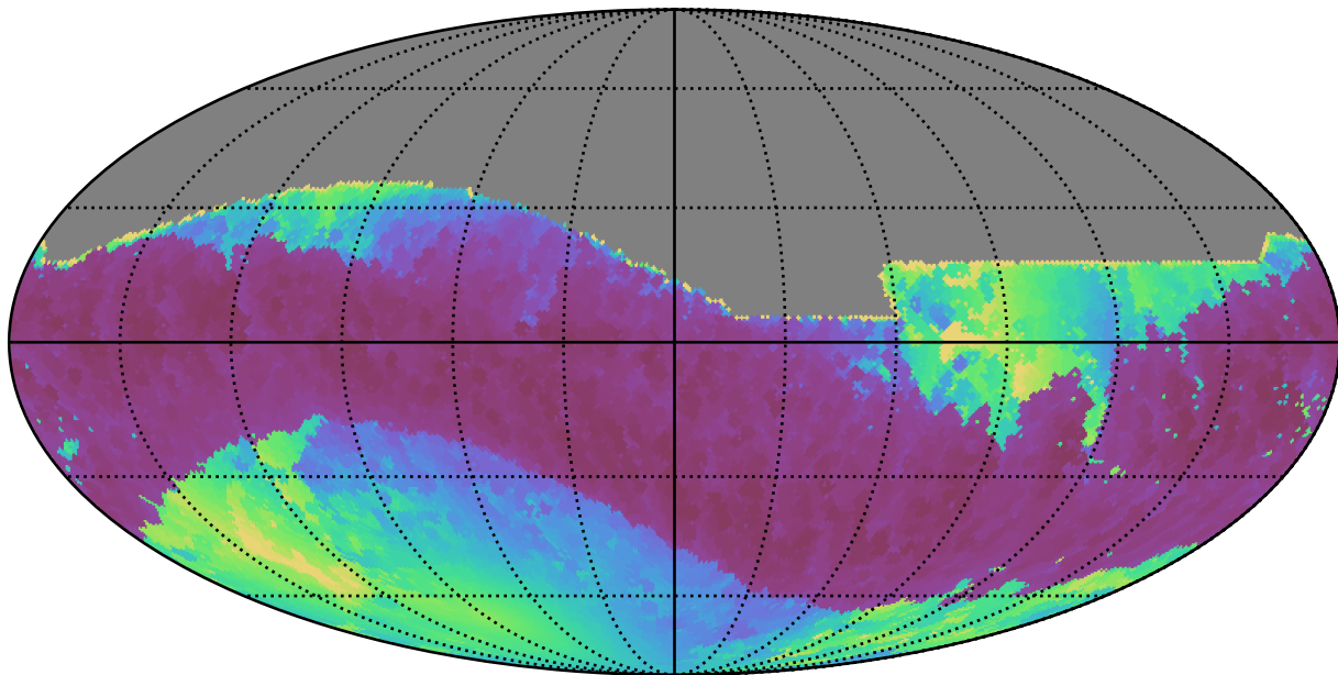
weather_cloudso20v3.4_10yrs All sky i band: Min solarElong
