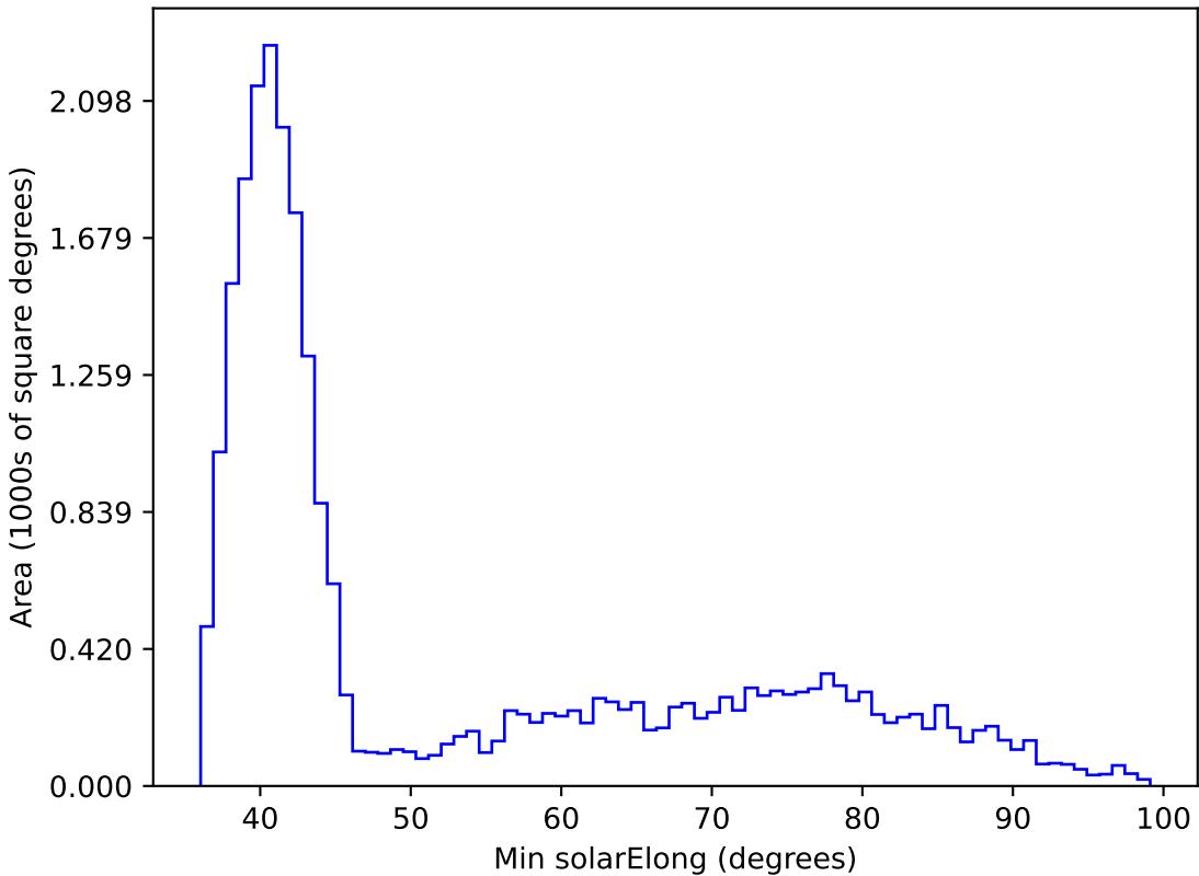
weather_cloudso20v3.4_10yrs All sky i band: Min solarElong
