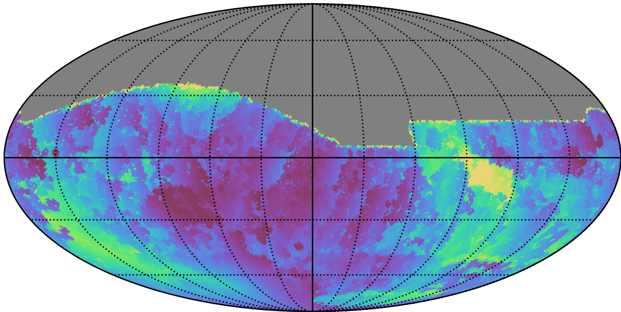
weather_cloudso20v3.4_10yrs All sky g band: Min solarElong
