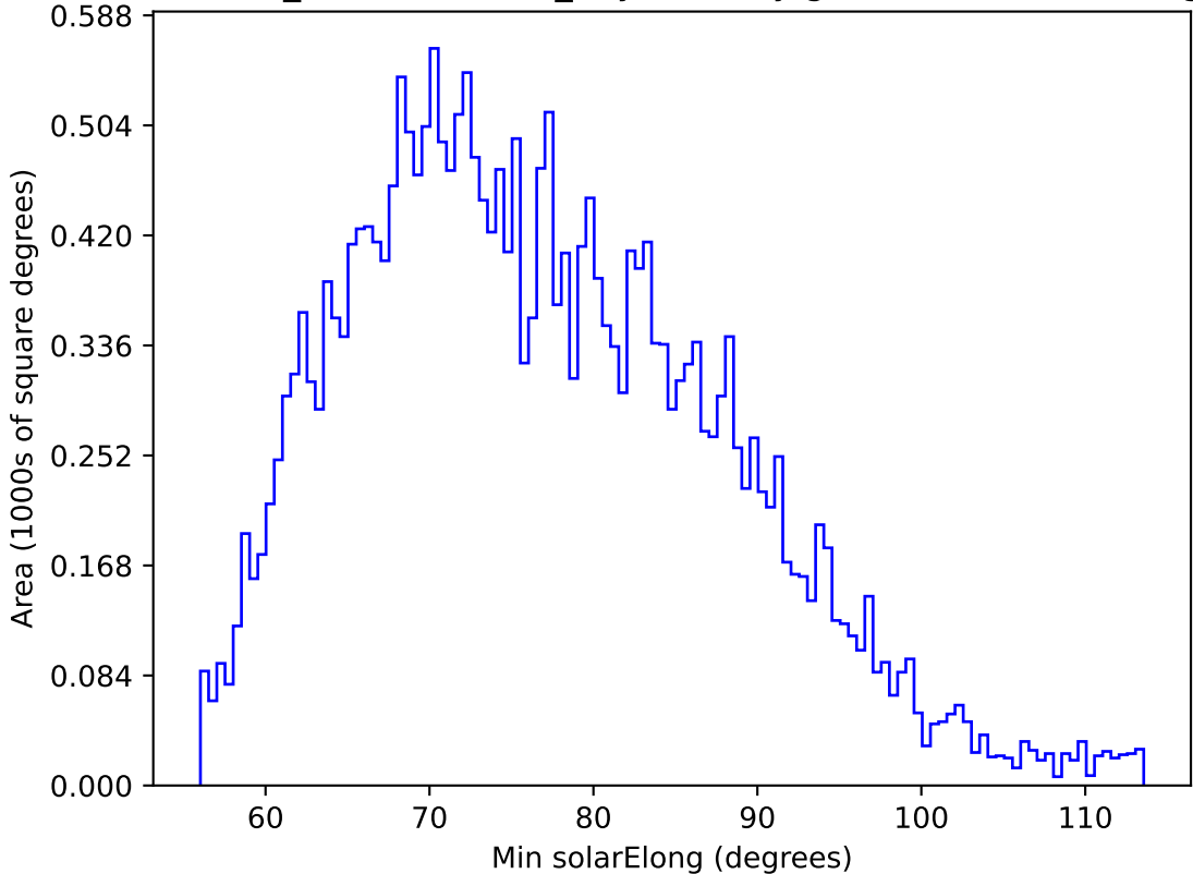
weather_cloudso20v3.4_10yrs All sky g band: Min solarElong
