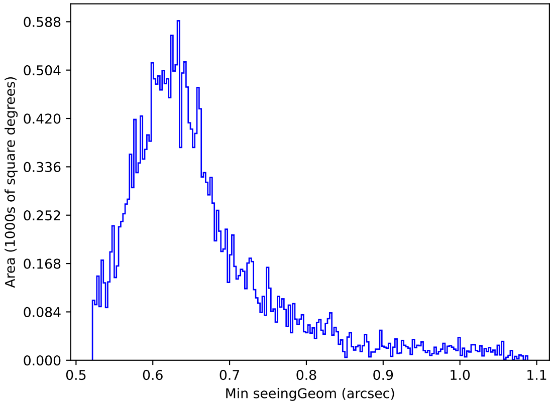
weather_cloudso20v3.4_10yrs Yr 1 z band: Min seeingGeom
