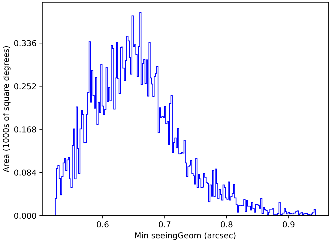
weather_cloudso20v3.4_10yrs Yr 1 y band: Min seeingGeom
