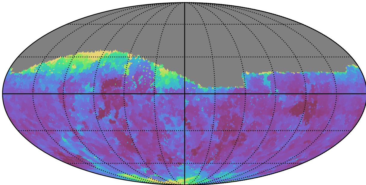
weather_cloudso20v3.4_10yrs Yr 1 r band: Min seeingGeom
