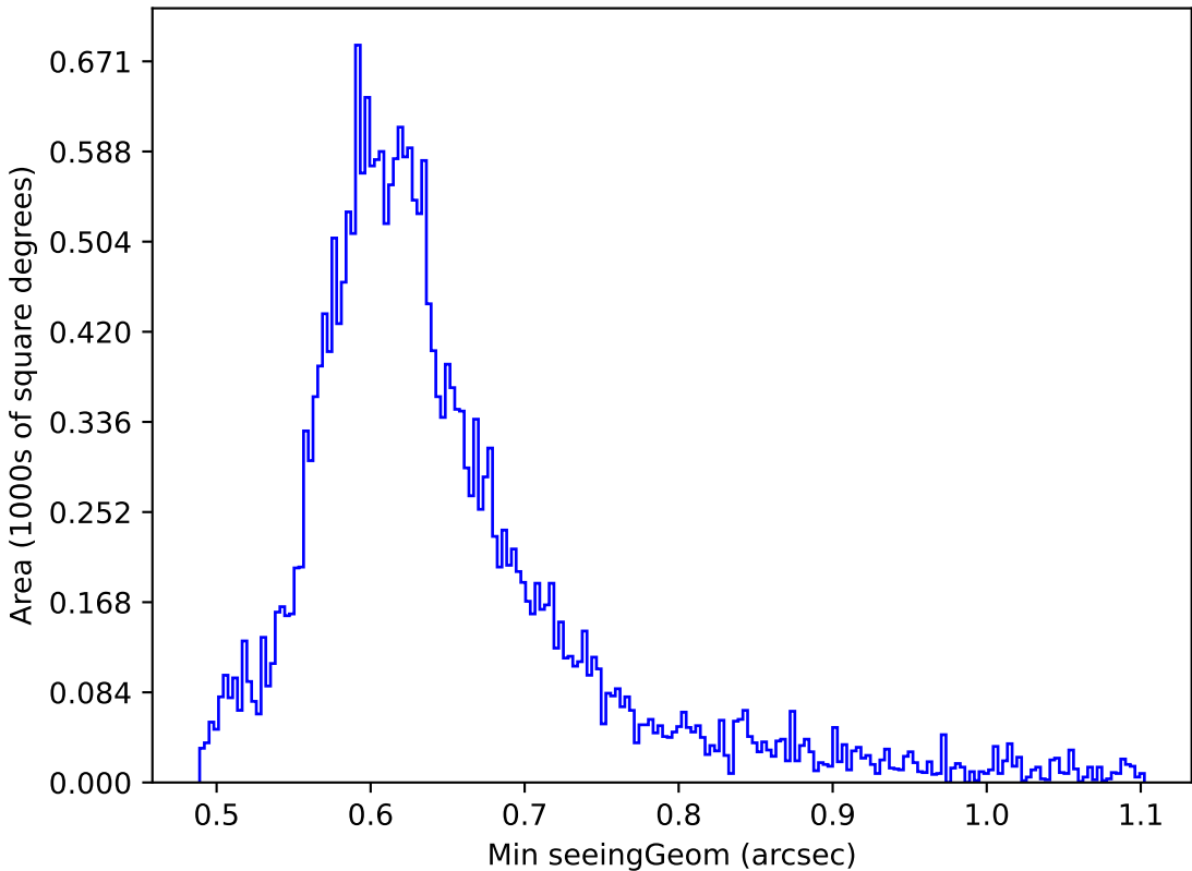
weather_cloudso20v3.4_10yrs Yr 1 r band: Min seeingGeom
