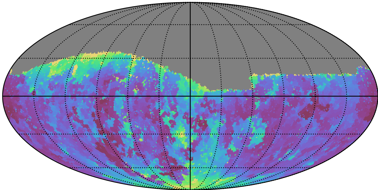
weather_cloudso20v3.4_10yrs Yr 1 g band: Min seeingGeom
