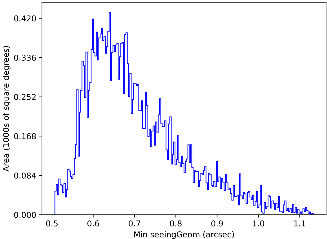
weather_cloudso20v3.4_10yrs Yr 1 g band: Min seeingGeom
