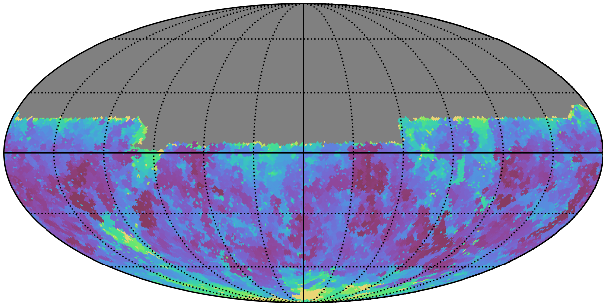
weather_cloudso20v3.4_10yrs Yr 1 y band: Min seeingEff
