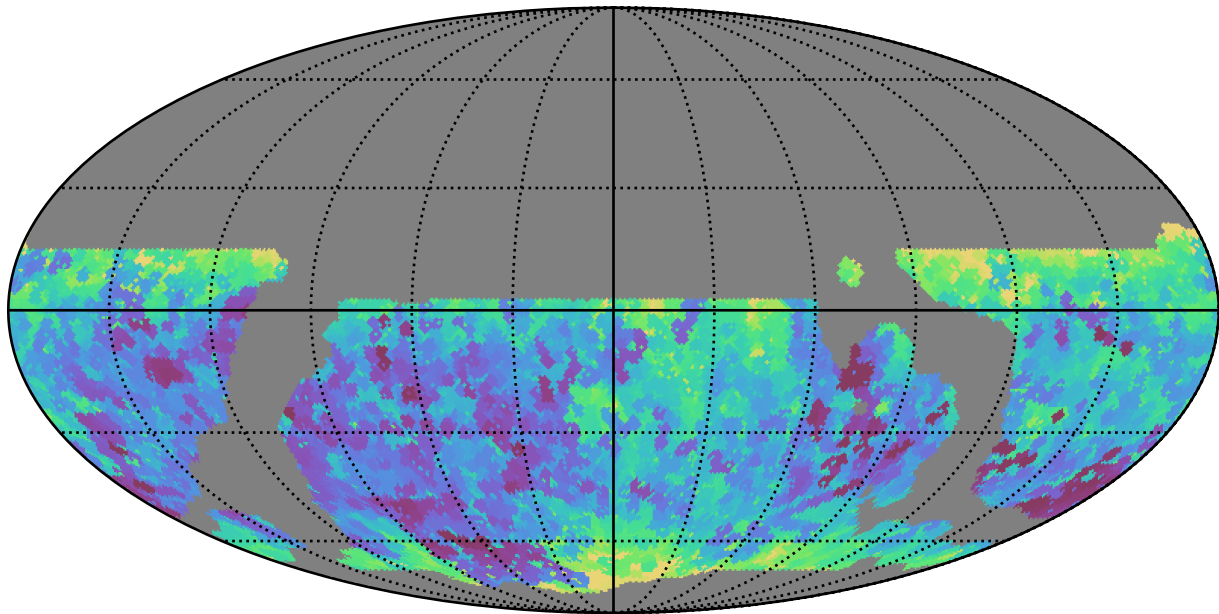
weather_cloudso20v3.4_10yrs WFD z band: Min seeingEff
