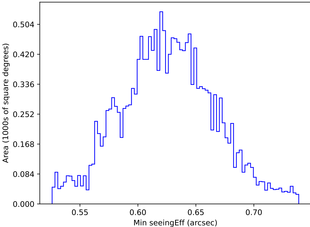
weather_cloudso20v3.4_10yrs WFD z band: Min seeingEff
