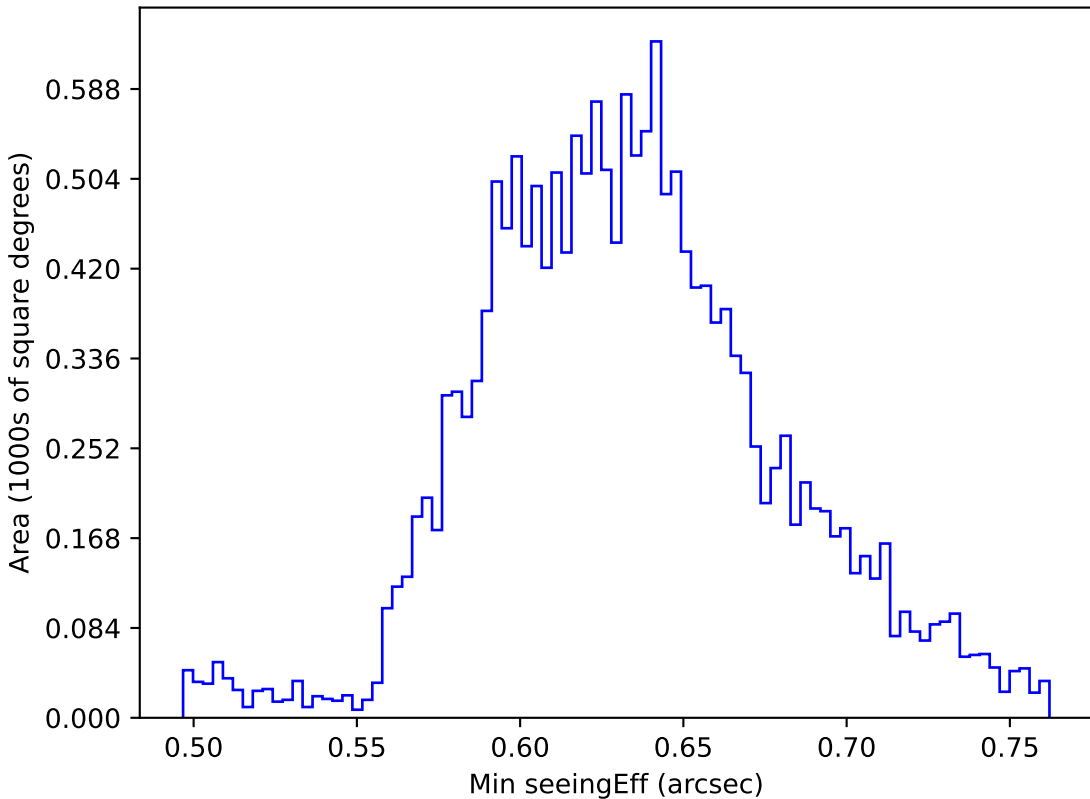
weather_cloudso20v3.4_10yrs WFD y band: Min seeingEff
