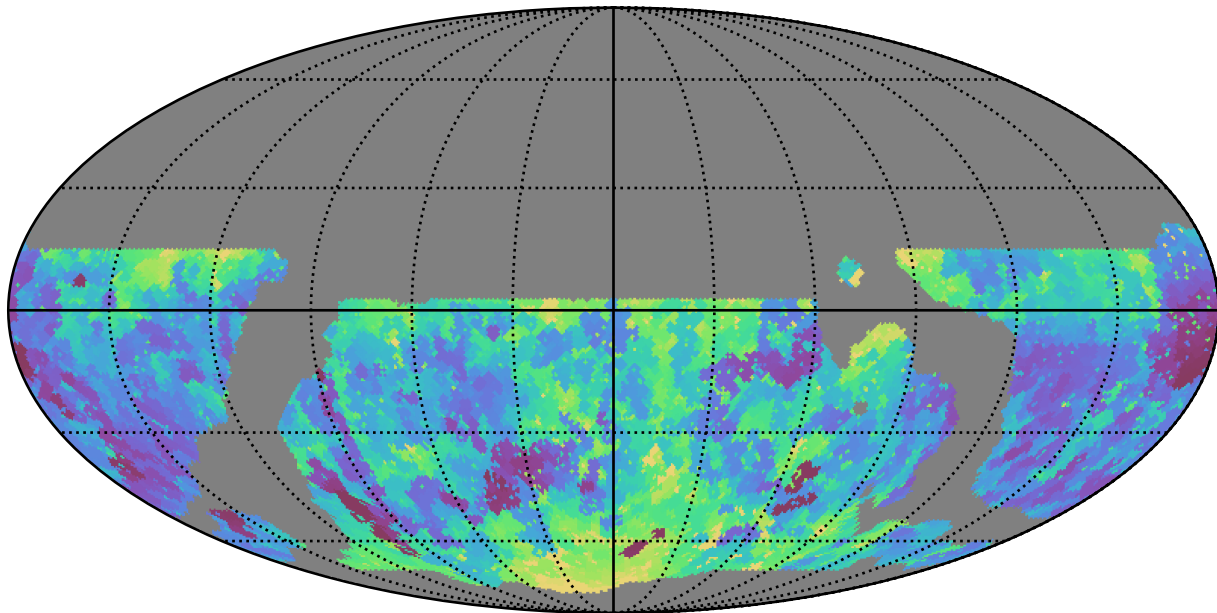
weather_cloudso20v3.4_10yrs WFD u band: Min seeingEff
