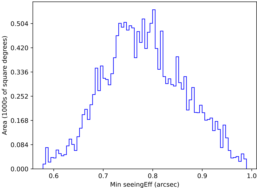
weather_cloudso20v3.4_10yrs WFD u band: Min seeingEff
