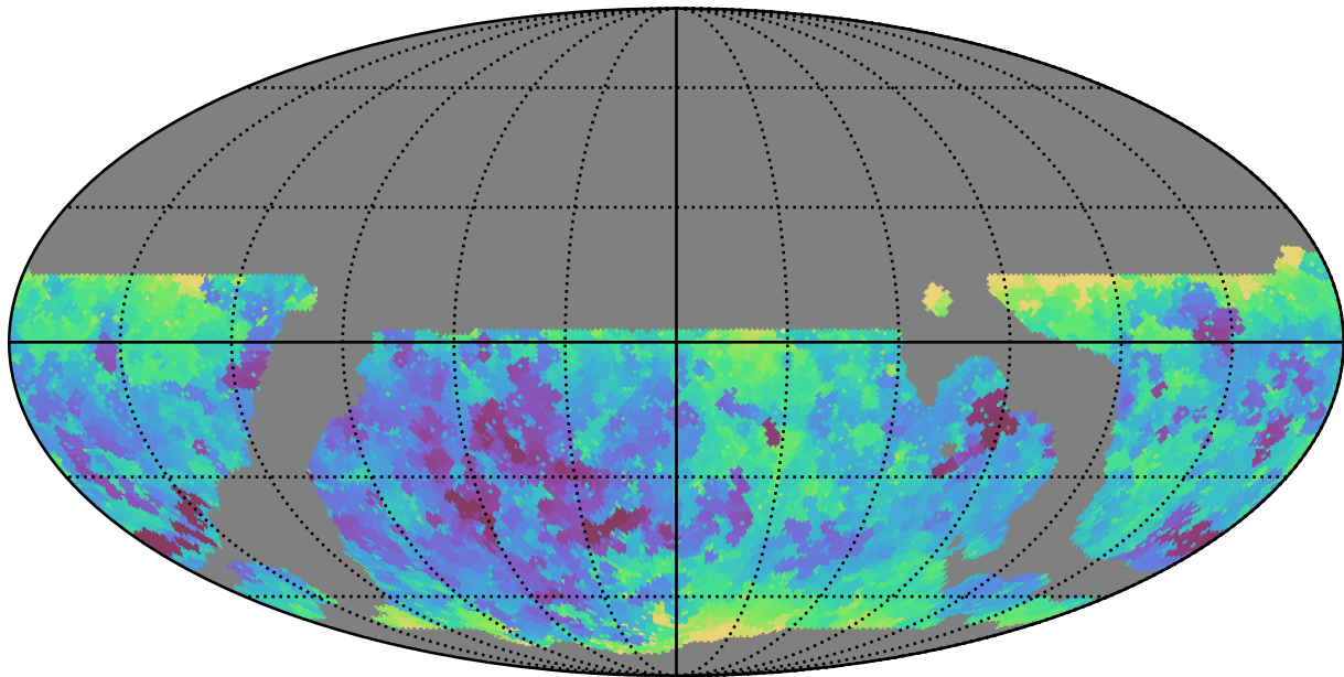
weather_cloudso20v3.4_10yrs WFD i band: Min seeingEff
