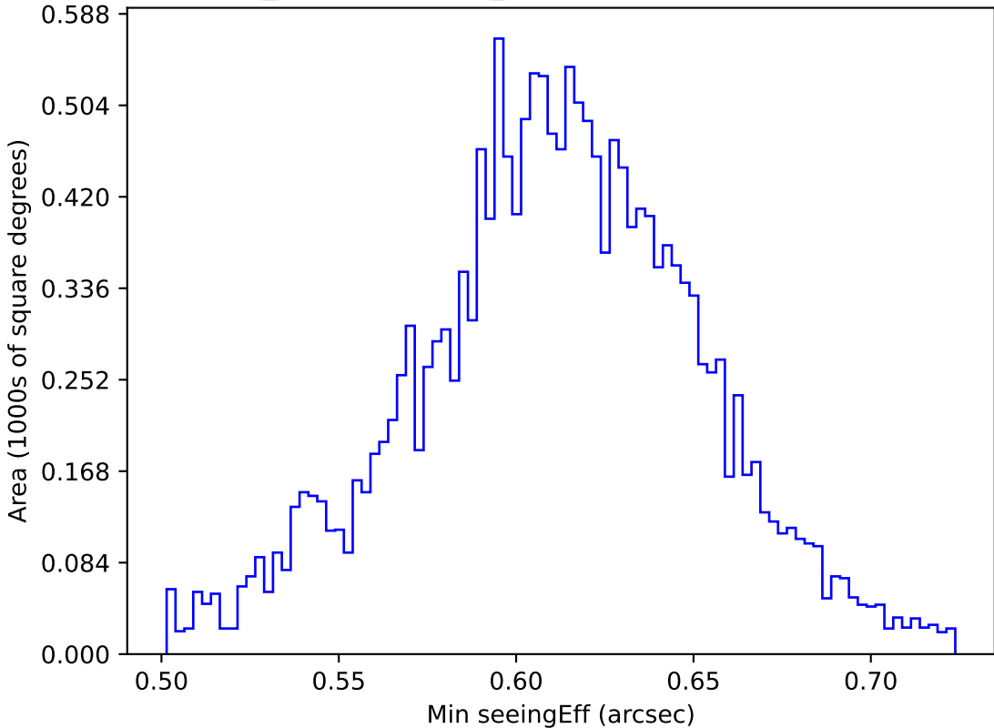
weather_cloudso20v3.4_10yrs WFD i band: Min seeingEff
