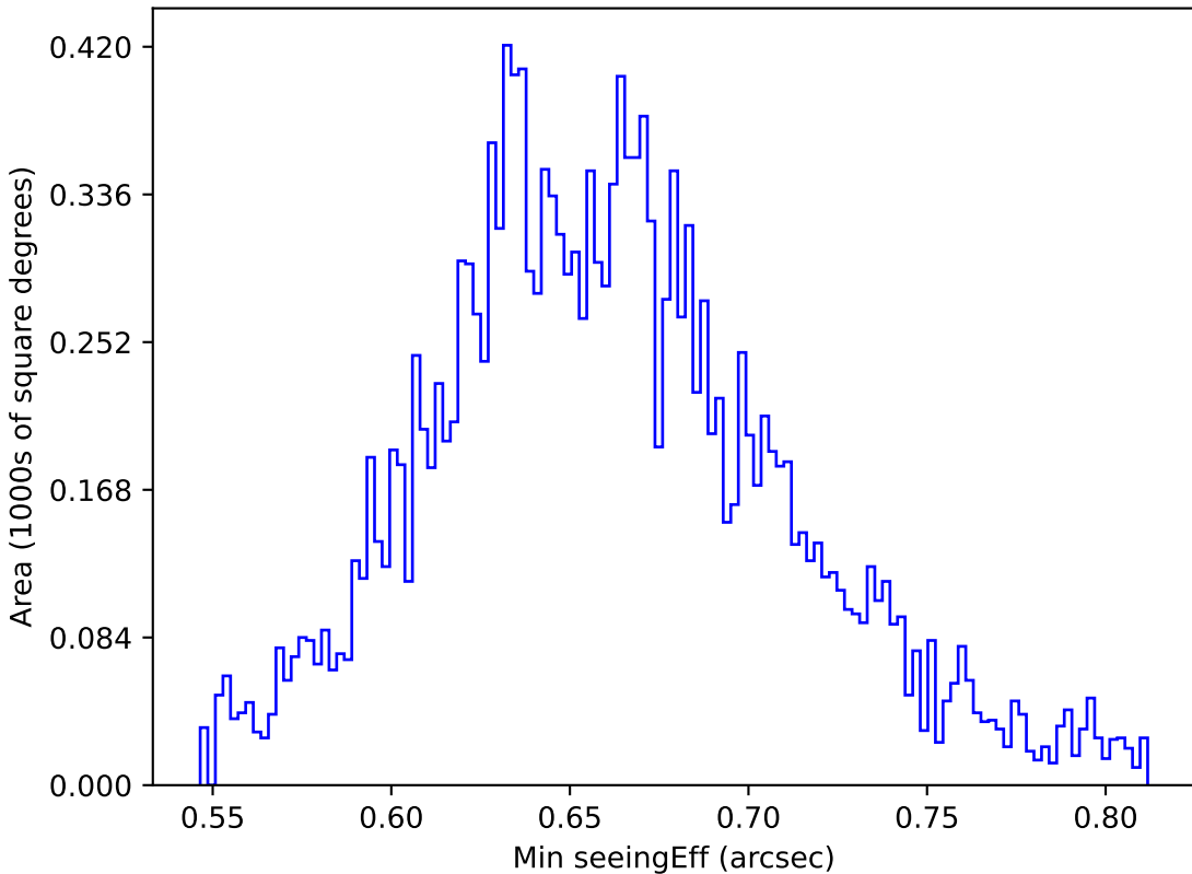
weather_cloudso20v3.4_10yrs WFD g band: Min seeingEff
