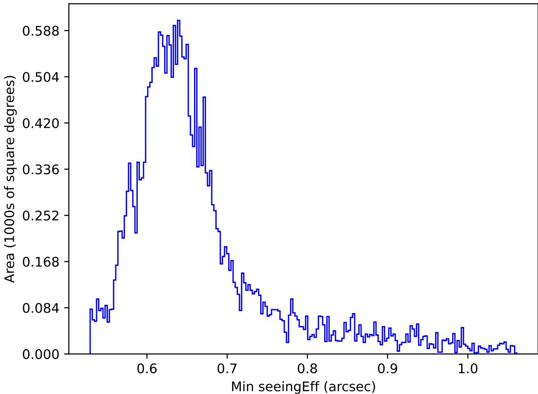
weather_cloudso20v3.4_10yrs All sky z band: Min seeingEff
