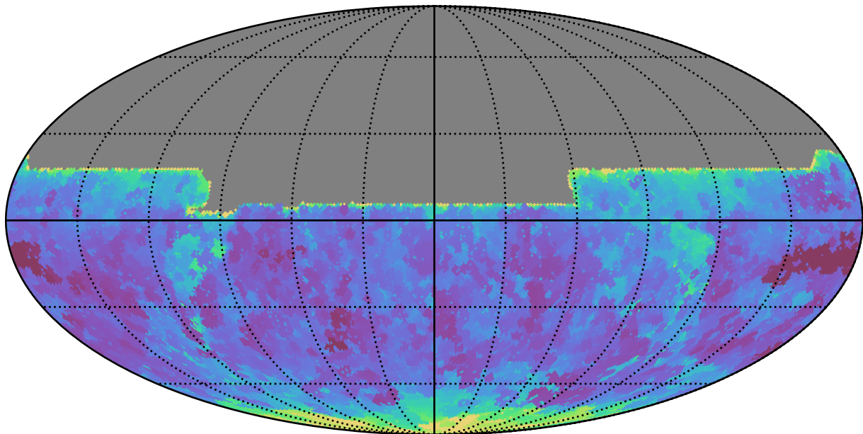
weather_cloudso20v3.4_10yrs All sky y band: Min seeingEff
