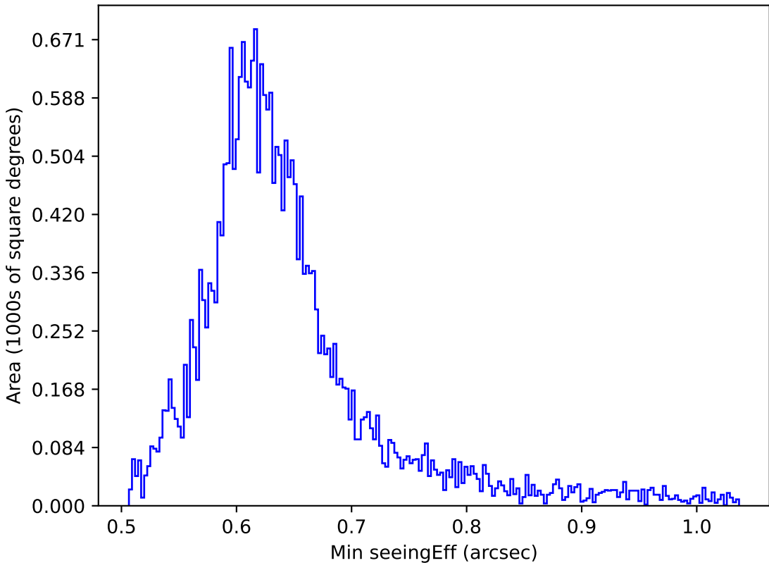
weather_cloudso20v3.4_10yrs All sky i band: Min seeingEff
