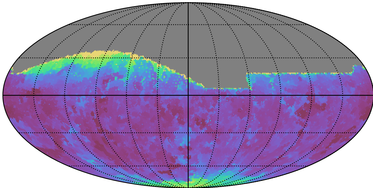
weather_cloudso20v3.4_10yrs All sky g band: Min seeingEff
