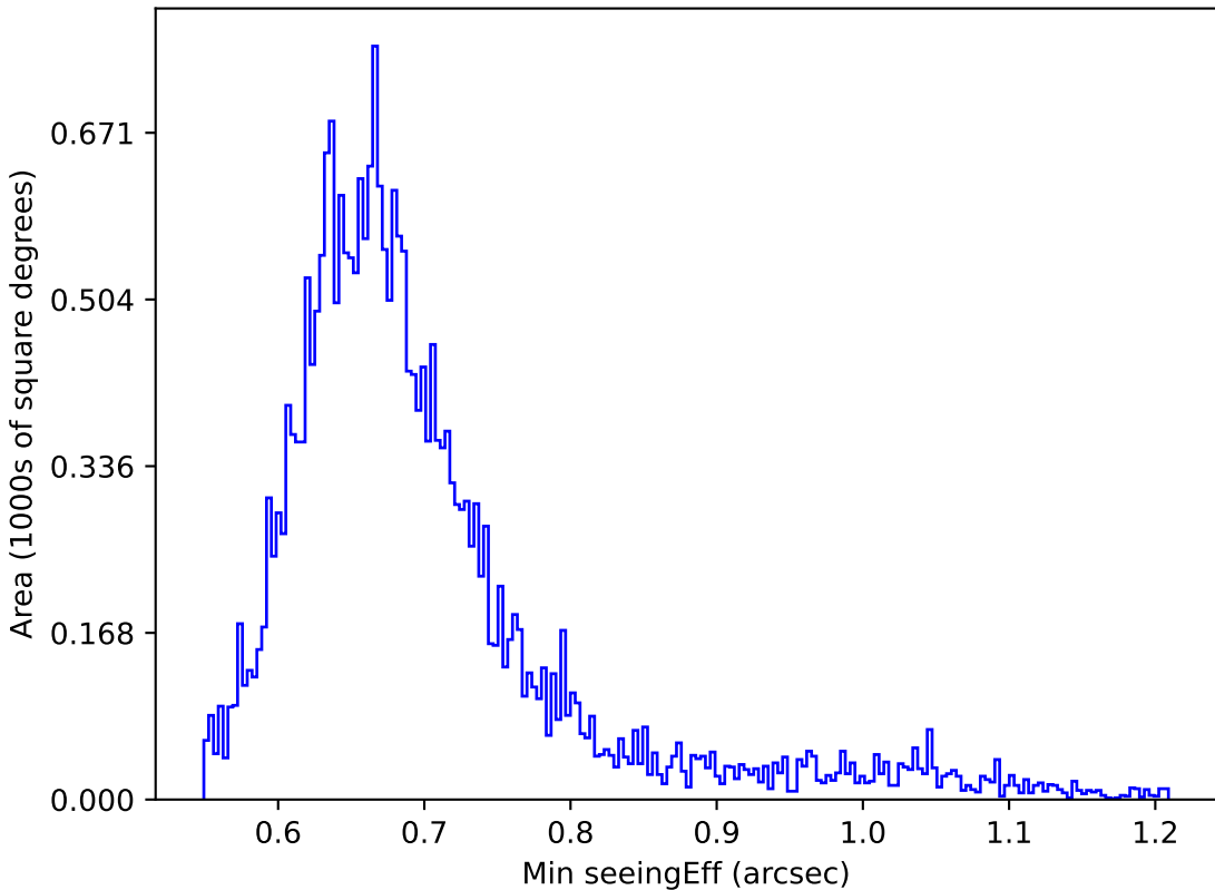
weather_cloudso20v3.4_10yrs All sky g band: Min seeingEff
