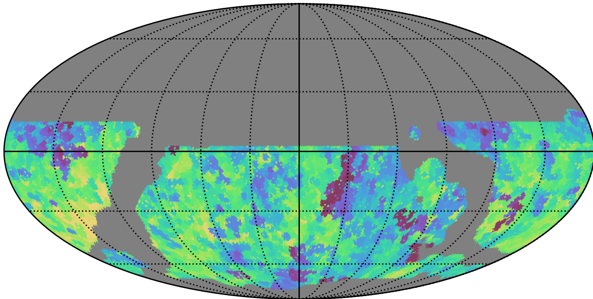
weather_cloudso20v3.4_10yrs WFD z band: Min saturation_mag
