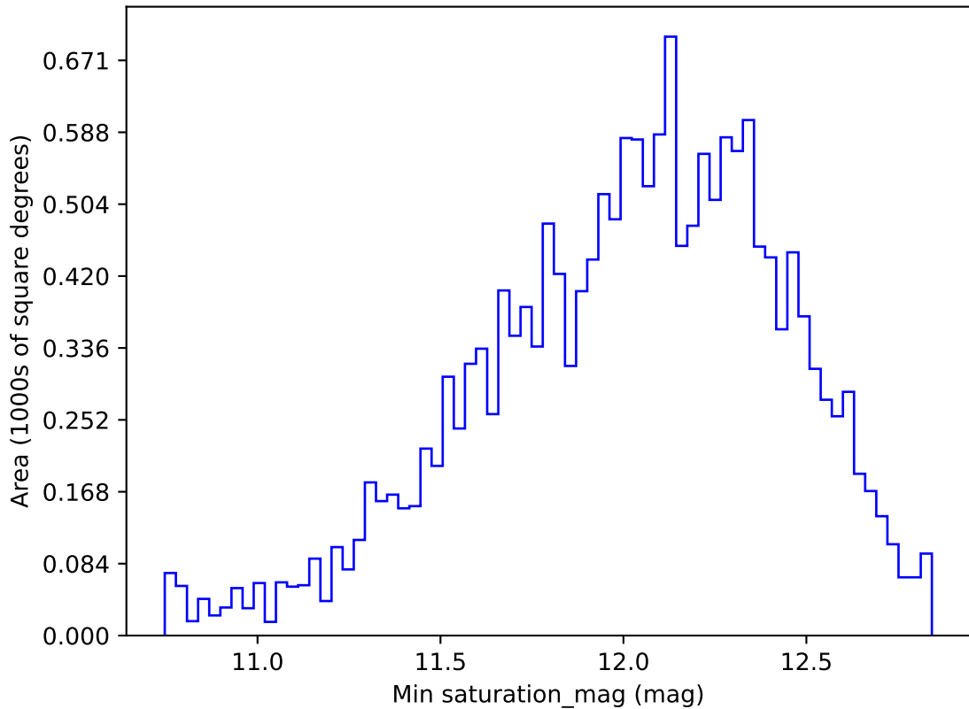
weather_cloudso20v3.4_10yrs WFD z band: Min saturation_mag
