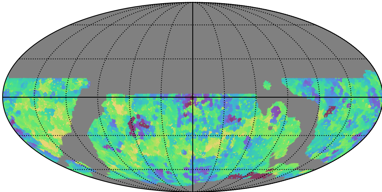
weather_cloudso20v3.4_10yrs WFD y band: Min saturation_mag
