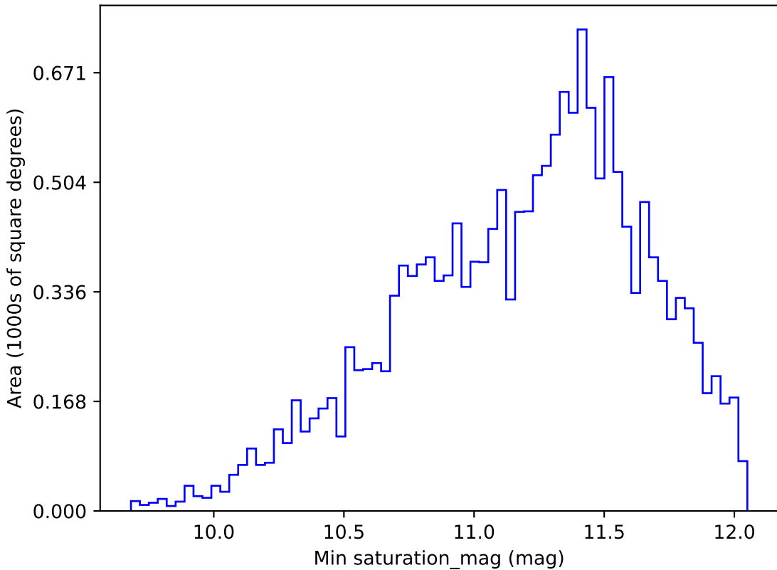
weather_cloudso20v3.4_10yrs WFD u band: Min saturation_mag
