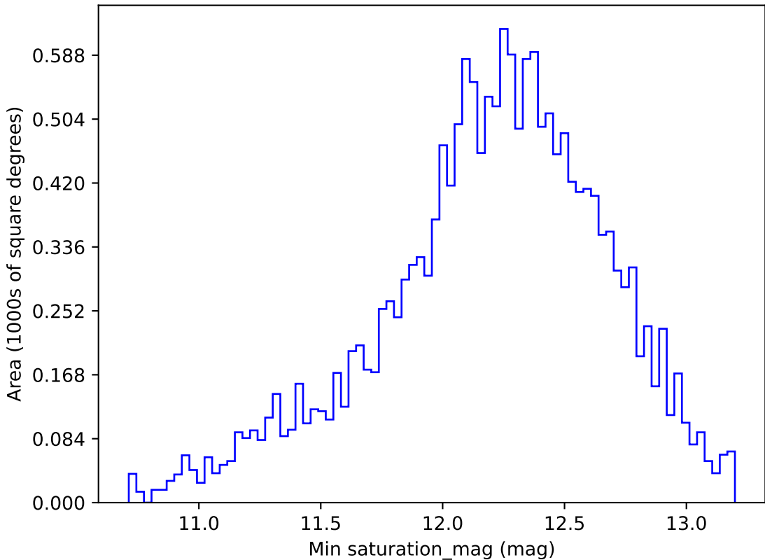
weather_cloudso20v3.4_10yrs WFD i band: Min saturation_mag
