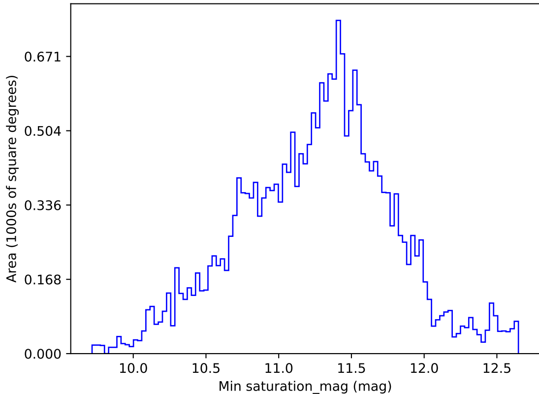
weather_cloudso20v3.4_10yrs All sky u band: Min saturation_mag
