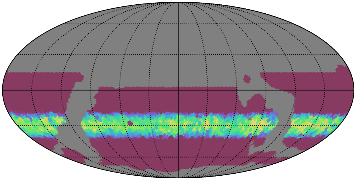
weather_cloudso20v3.4_10yrs WFD z band: Min normairmass
