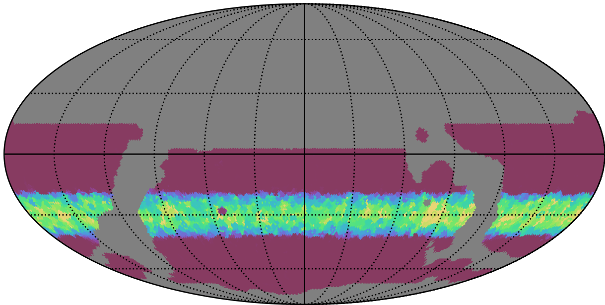
weather_cloudso20v3.4_10yrs WFD y band: Min normairmass
