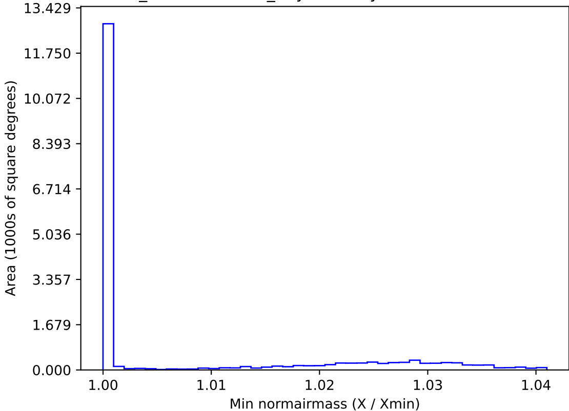
weather_cloudso20v3.4_10yrs WFD y band: Min normairmass
