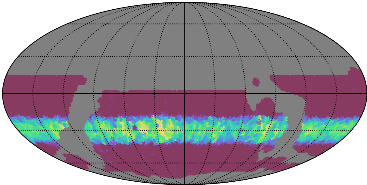
weather_cloudso20v3.4_10yrs WFD u band: Min normairmass
