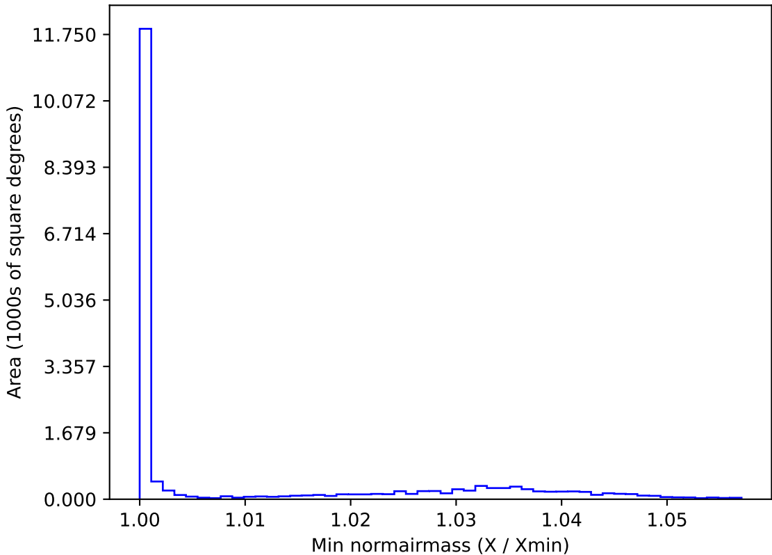
weather_cloudso20v3.4_10yrs WFD u band: Min normairmass
