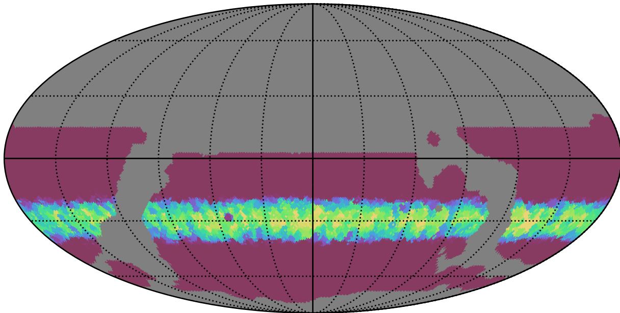
weather_cloudso20v3.4_10yrs WFD r band: Min normairmass
