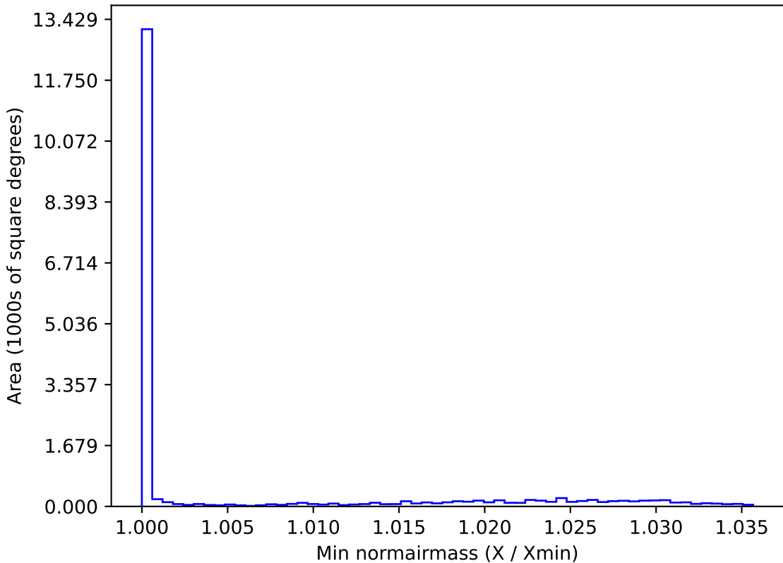
weather_cloudso20v3.4_10yrs WFD r band: Min normairmass
