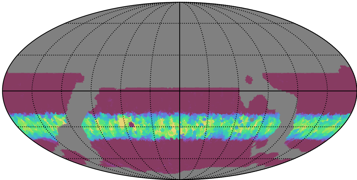
weather_cloudso20v3.4_10yrs WFD g band: Min normairmass
