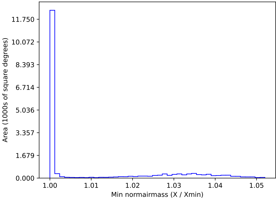
weather_cloudso20v3.4_10yrs WFD g band: Min normairmass
