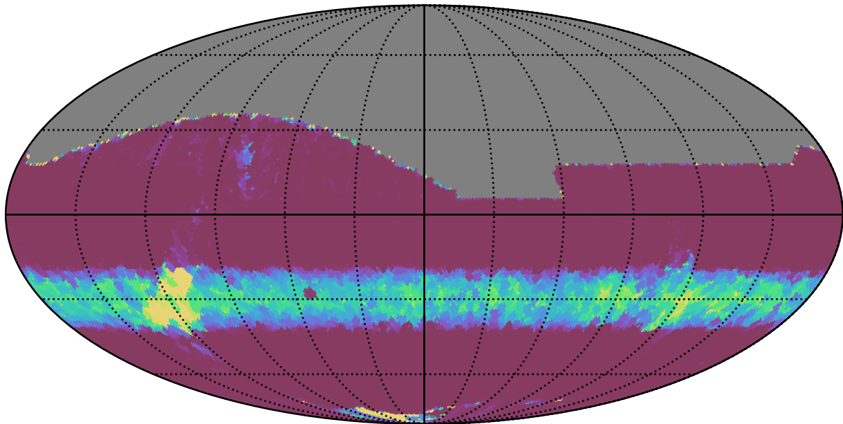
weather_cloudso20v3.4_10yrs All sky z band: Min normairmass
